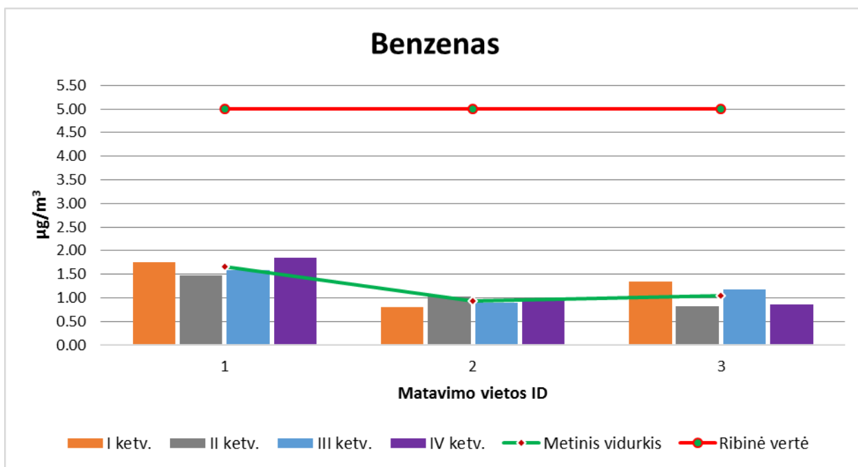
10 pav. Benzeno koncentracijų pasiskirstymai Kupiškio rajone pagal nustatytą matavimo vietos ID
