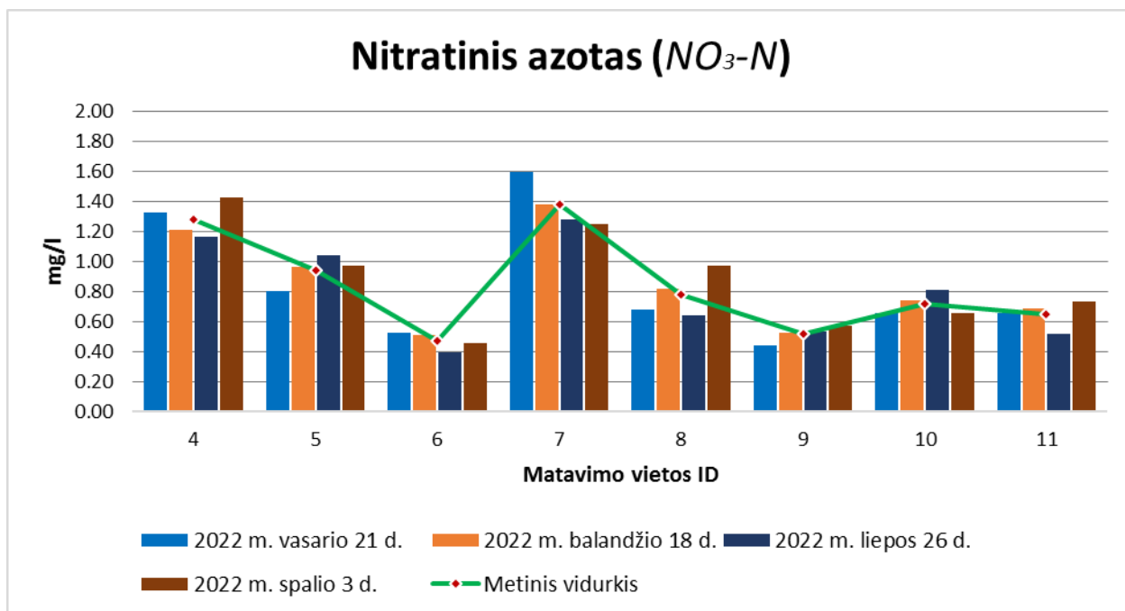
19 pav. Kupiškio rajono savivaldybės upių nitratinio azoto ( NO_3-N ) tyrimo rezultatų vizualizacija. (Ribinė vertė 9 mg/l grafike neatvaizduojama, nes gautos nitratinio azoto koncentracijų vertės ženkliai mažesnės)
