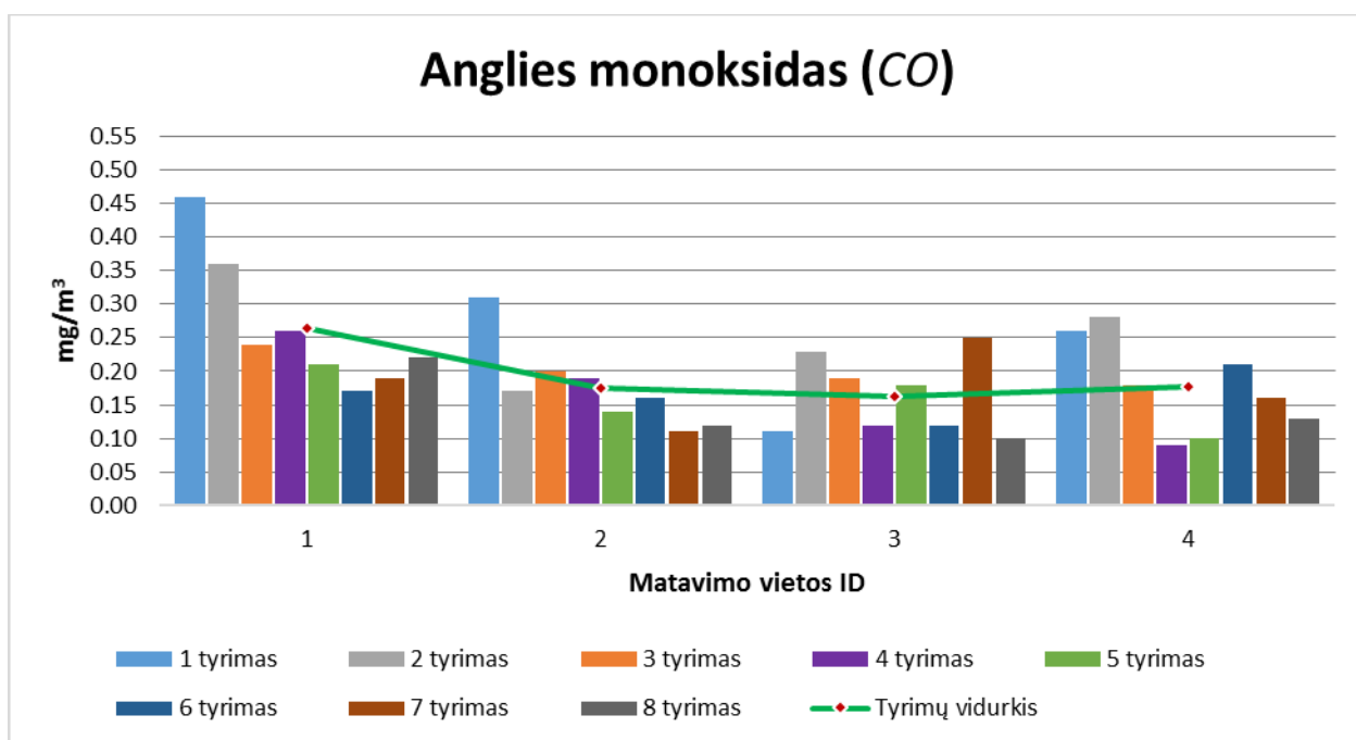
7 pav. CO koncentracijų pasiskirstymai Kupiškio rajone pagal nustatytą matavimo vietos ID. (Ribinė vertė 10 \text{ mg}/\text{m}^3 grafike neatvaizduojama, nes gautos anglies monoksido koncentracijos ženkliai mažesnės už ribinę vertę)
