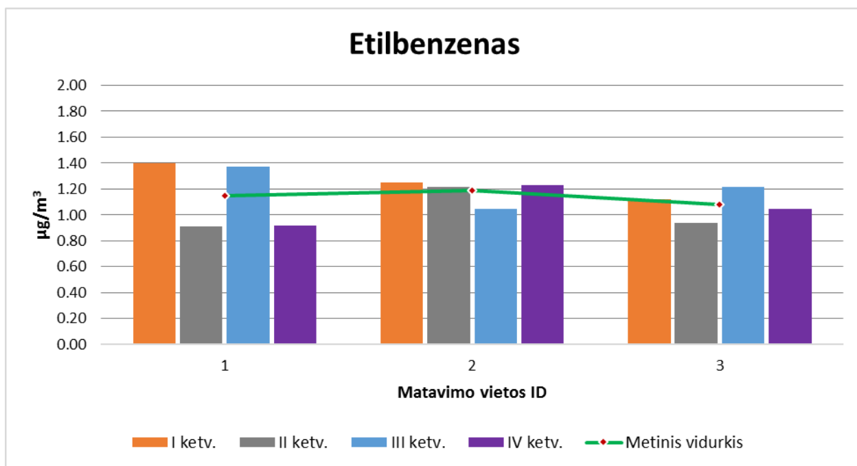
12 pav. Etilbenzeno koncentracijų pasiskirstymai Kupiškio rajone pagal nustatytą matavimo vietos ID. (Ribinė vertė 20 \mu\text{g}/\text{m}^3 grafike neatvaizduojama, nes gautos etilbenzeno koncentracijos ženkliai mažesnės už ribinę vertę)
