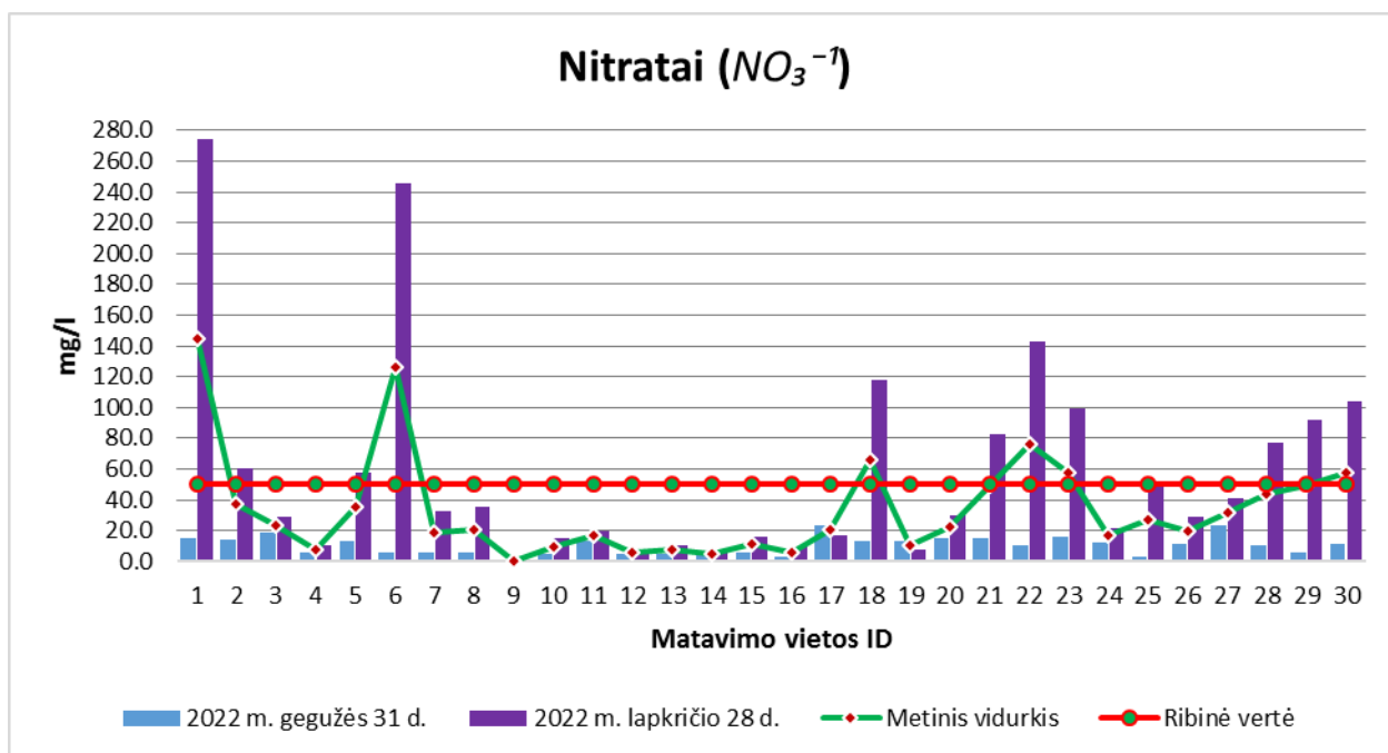
40 pav. Nitratų koncentracijų vizualizacija Kupiškio rajono požeminiame vandenyje
