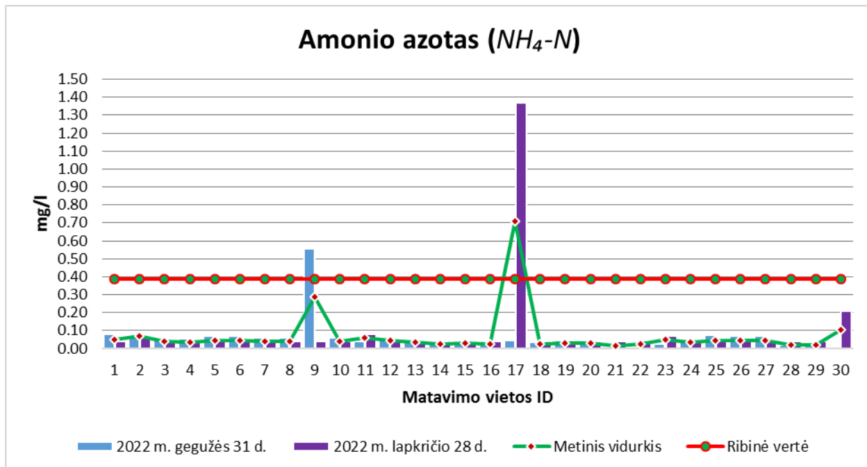
41 pav. Amonio azoto koncentracijų vizualizacija Kupiškio rajono požeminiame vandenyje
