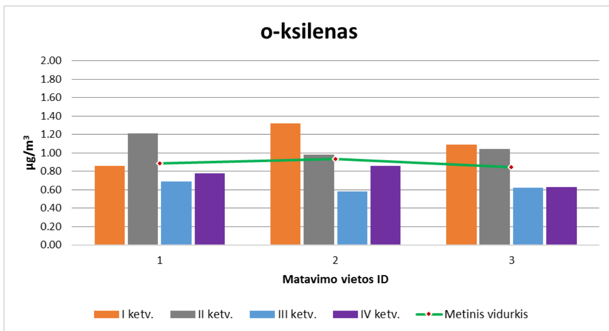
14 pav. o-ksileno koncentracijų pasiskirstymai Kupiškio rajone pagal nustatytą matavimo vietos ID. (Ribinė vertė 200 \mu\text{g}/\text{m}^3 grafike neatvaizduojama, nes gautos o-ksileno koncentracijos ženkliai mažesnės už ribinę vertę)
