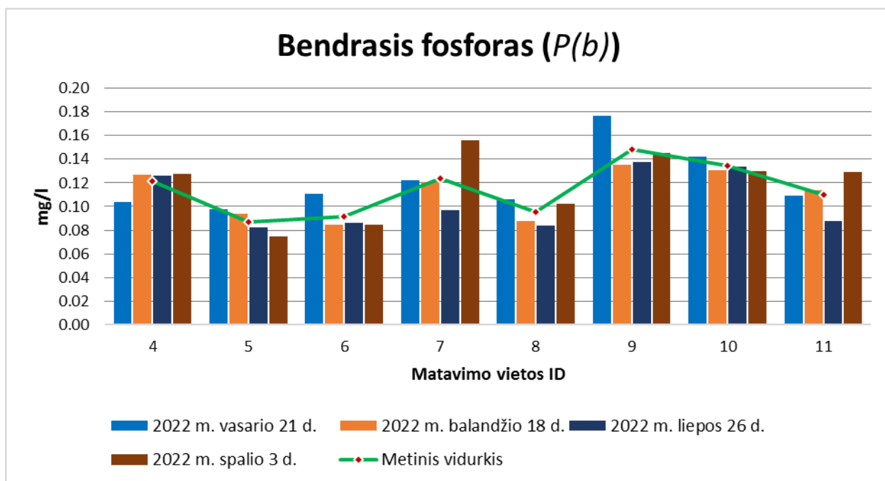
20 pav. Kupiškio rajono savivaldybės upių bendrojo foforo tyrimo rezultatų vizualizacija. (Ribinė vertė 2 mg/l grafike neatvaizduojama, nes gautos P_b koncentracijos ženkliai mažesnės už ribinę vertę)
