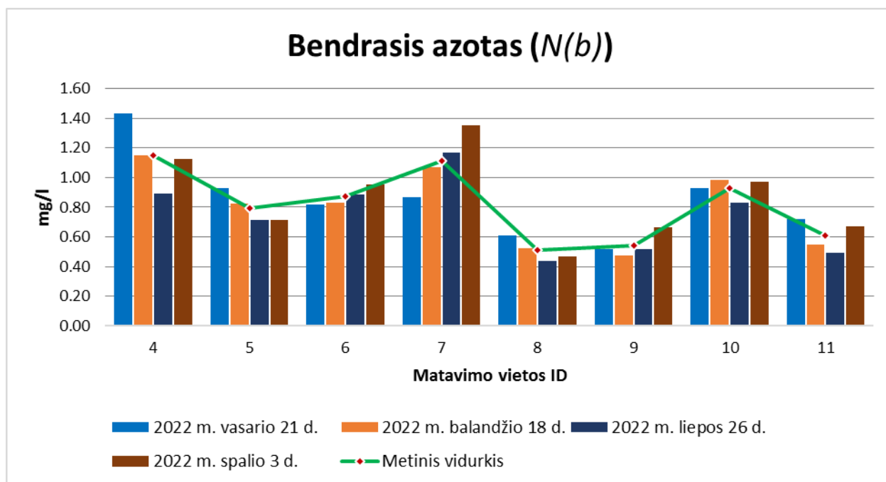
17 pav. Kupiškio rajono savivaldybės upių bendrojo azoto tyrimo rezultatų vizualizacija. (Ribinė vertė 12 mg/l grafike neatvaizduojama, nes gautos N b koncentracijos ženkliai mažesnės už ribinę vertę)
