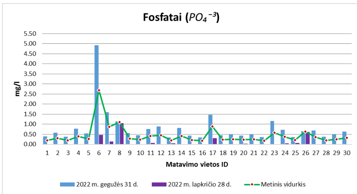
44 pav. fosfatų koncentracijų vizualizacija Kupiškio rajono požeminiame vandenyje
