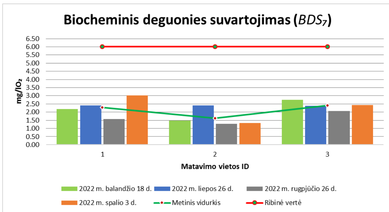
25 pav. Kupiškio rajono savivaldybės ežerų ir tvenkinio vandens BDS_7 tyrimo rezultatų vizualizacija.
