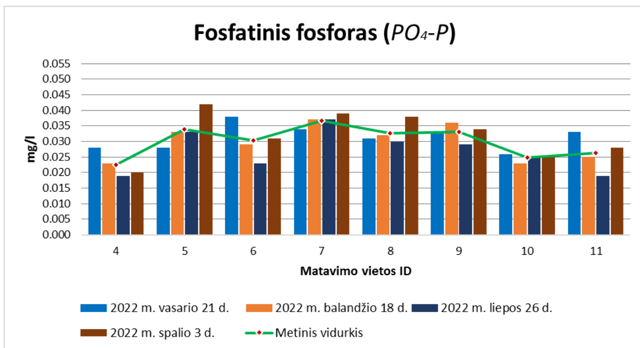
21 pav. Kupiškio rajono savivaldybės upių fosfatinio fosforo ( PO_4-P ) tyrimo rezultatų vizualizacija.
