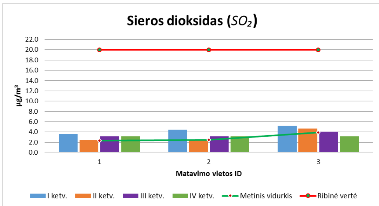
9 pav. SO_2 koncentracijų pasiskirstymai Kupiškio rajone pagal nustatytą matavimo vietos ID
