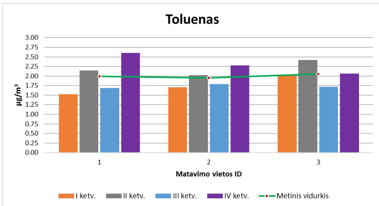
11 pav. Tolueno koncentracijų pasiskirstymai Kupiškio rajone pagal nustatytą matavimo vietos ID.
