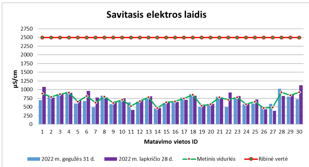
39 pav. Savitojo elektros laidžio koncentracijų vizualizacija Kupiškio rajono požeminiame vandenyje
