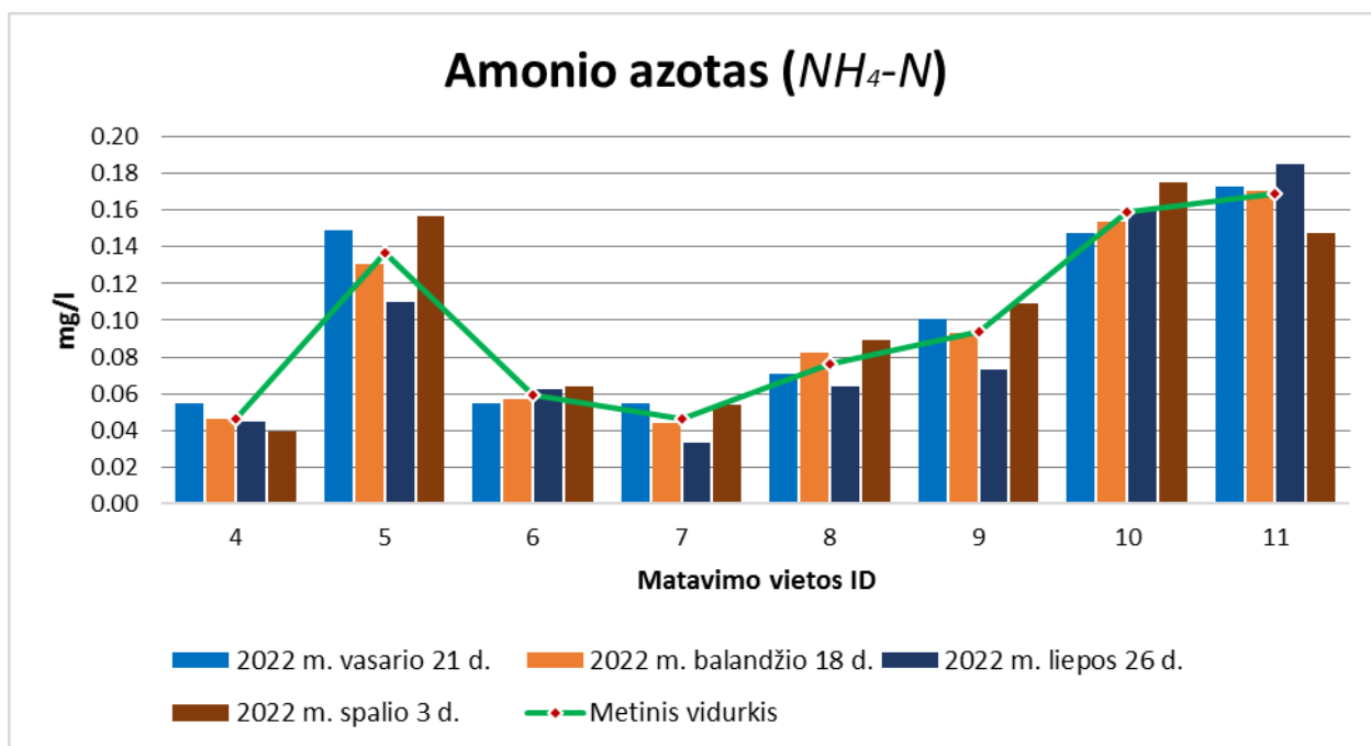
18 pav. Kupiškio rajono savivaldybės upių amonio azoto ( NH_4-N ) tyrimo rezultatų vizualizacija. (Ribinė vertė 2 mg/l grafike neatvaizduojama, nes gautos amonio azoto koncentracijos ženkliai mažesnės už ribinę vertę)
