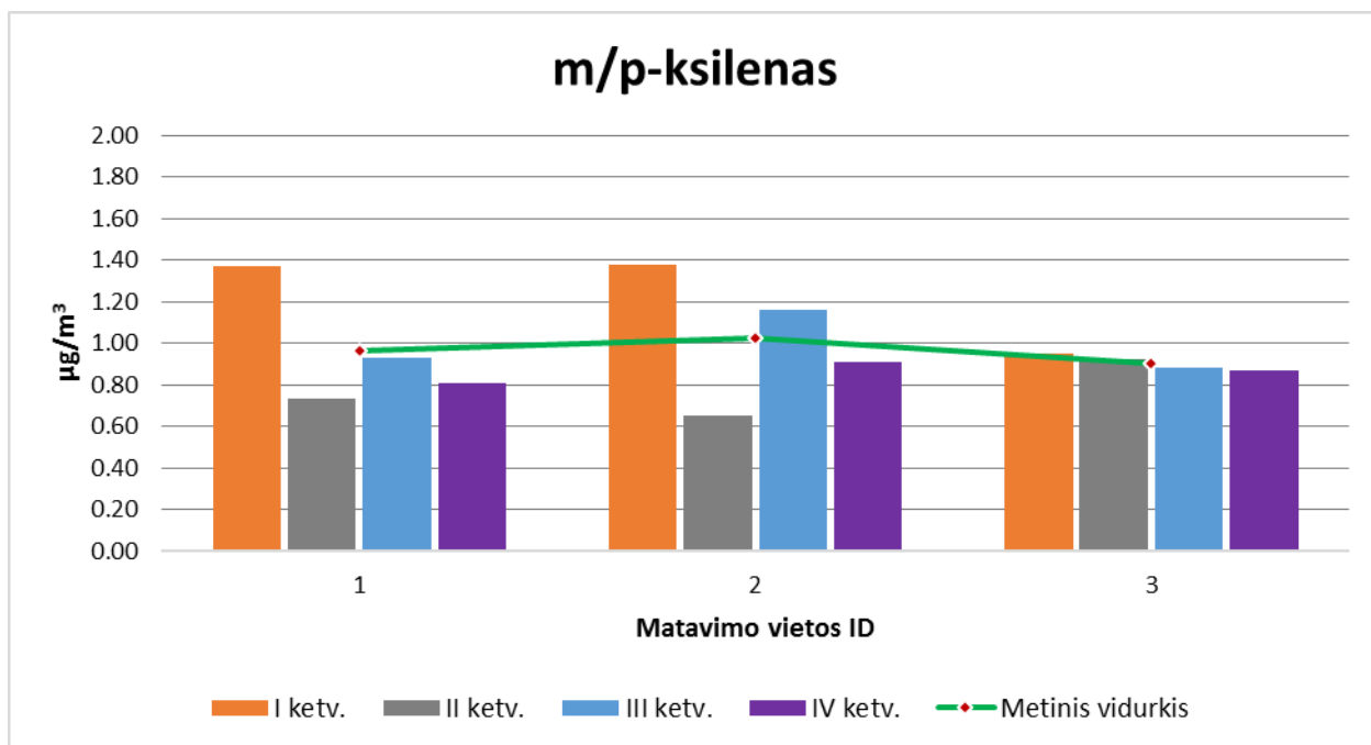
13 pav. m/p-ksileno koncentracijų pasiskirstymai Kupiškio rajone pagal nustatytą matavimo vietos ID. (Ribinė vertė 200 \mu\text{g}/\text{m}^3 grafike neatvaizduojama, nes gautos m/p-ksileno koncentracijos ženkliai mažesnės už ribinę vertę)
