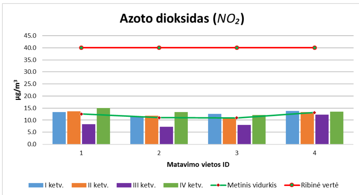
8 pav. NO_2 koncentracijų pasiskirstymai Kupiškio rajone pagal nustatytą matavimo vietos ID
