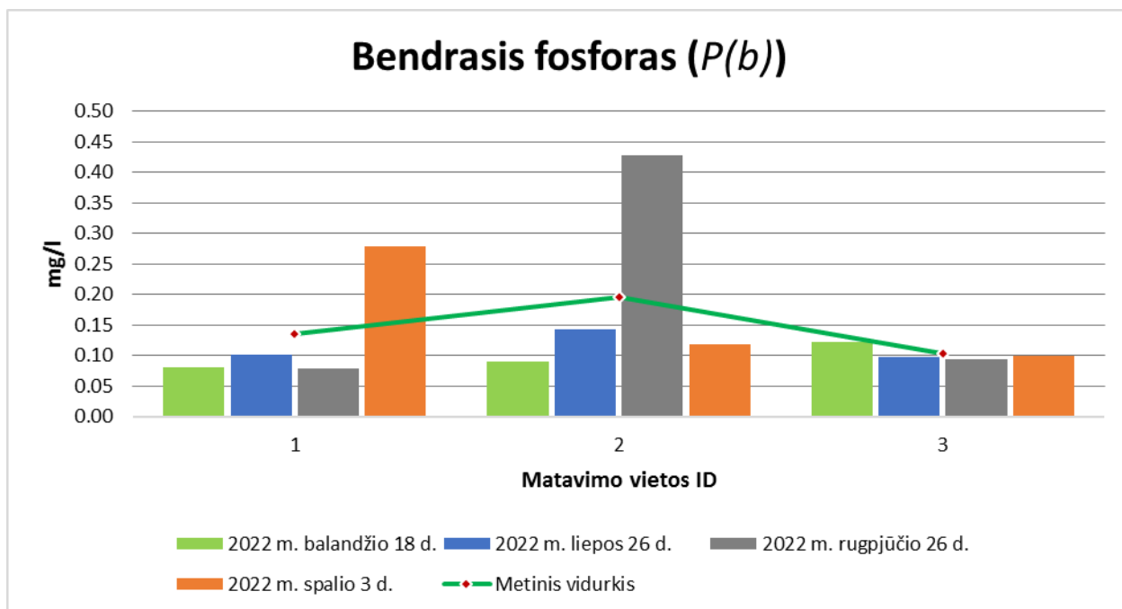
24 pav. Kupiškio rajono savivaldybės ežerų ir tvenkinio vandens bendrojo fosforo tyrimo rezultatų vizualizacija. (Ribinė vertė 1,6 mg/l grafike neatvaizduojama, nes gautos P_b koncentracijos ženkliai mažesnės už ribinę vertę)
