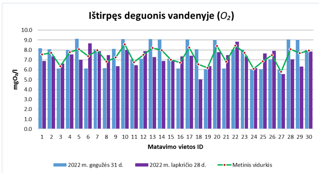
37 pav. Ištirpusio deguonies koncentracijų vizualizacija Kupiškio rajono požeminiame vandenyje
