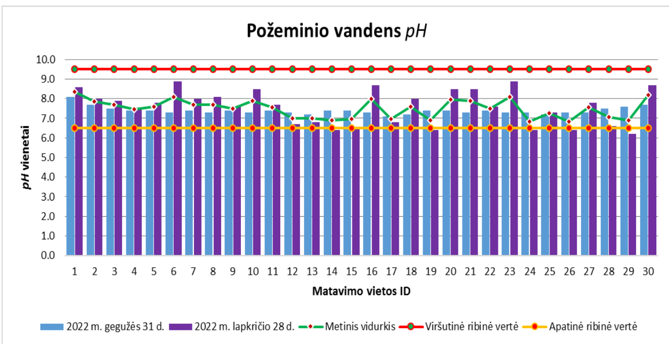
38 pav. pH koncentracijų vizualizacija Kupiškio rajono požeminiame vandenyje
