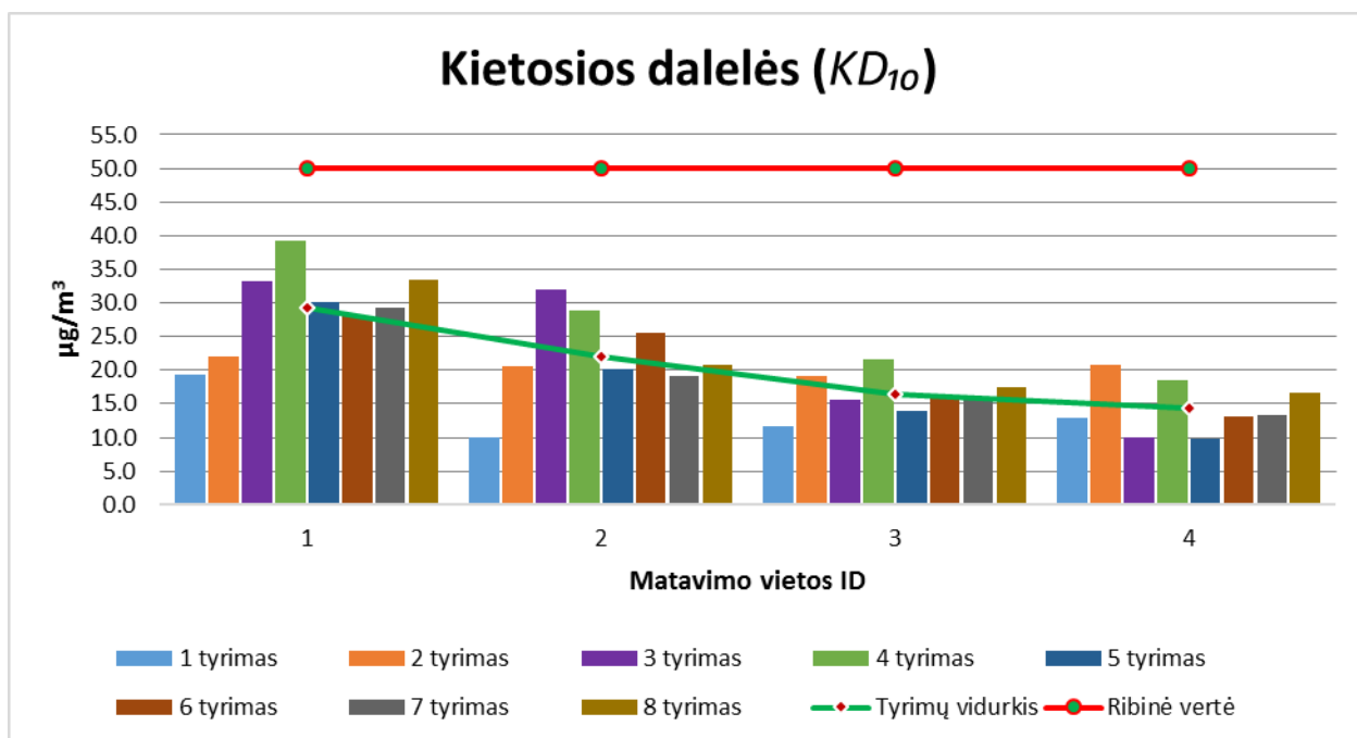
6 pav. KD_{10} koncentracijų pasiskirstymai Kupiškio rajone pagal nustatytą matavimo vietos ID
