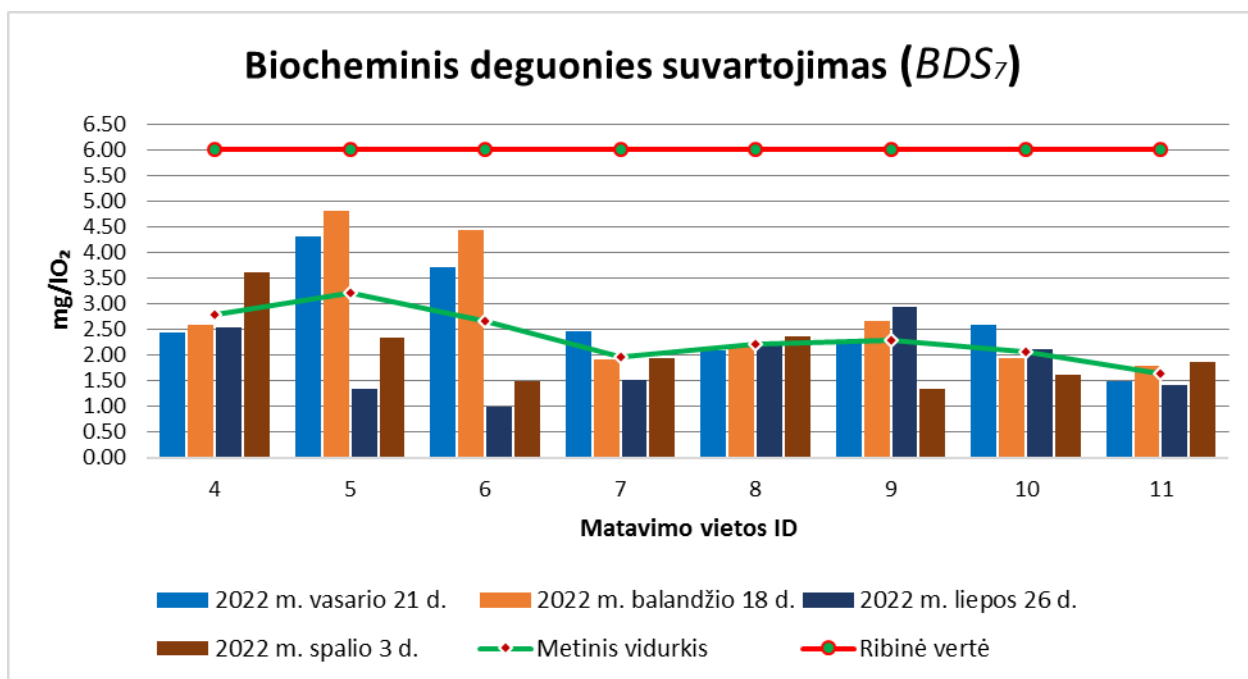
22 pav. Kupiškio rajono savivaldybės upių BDS_7 tyrimo rezultatų vizualizacija.
