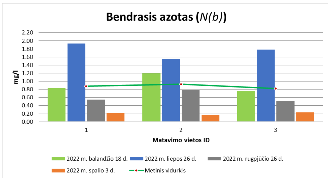
23 pav. Kupiškio rajono savivaldybės ežerų ir tvenkinio vandens bendrojo azoto tyrimo rezultatų vizualizacija. (Ribinė vertė 12 mg/l grafike neatvaizduojama, nes gautos N_b koncentracijos ženkliai mažesnės už ribinę vertę)
