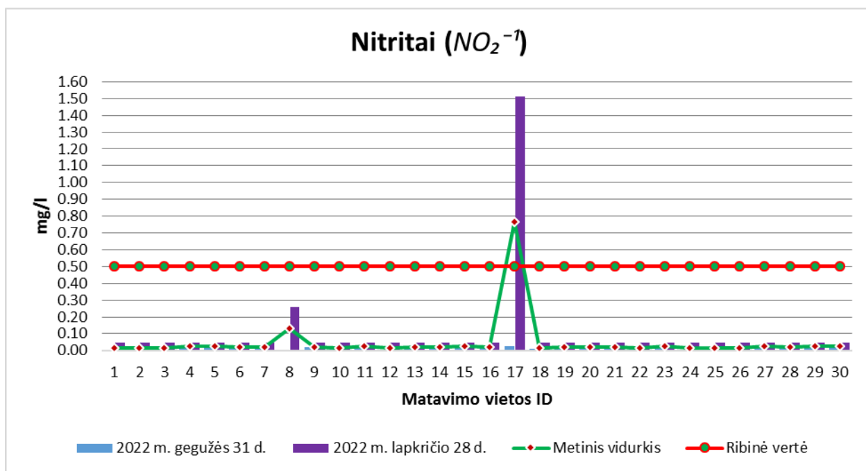
42 pav. Nitritų koncentracijų vizualizacija Kupiškio rajono požeminiame vandenyje
