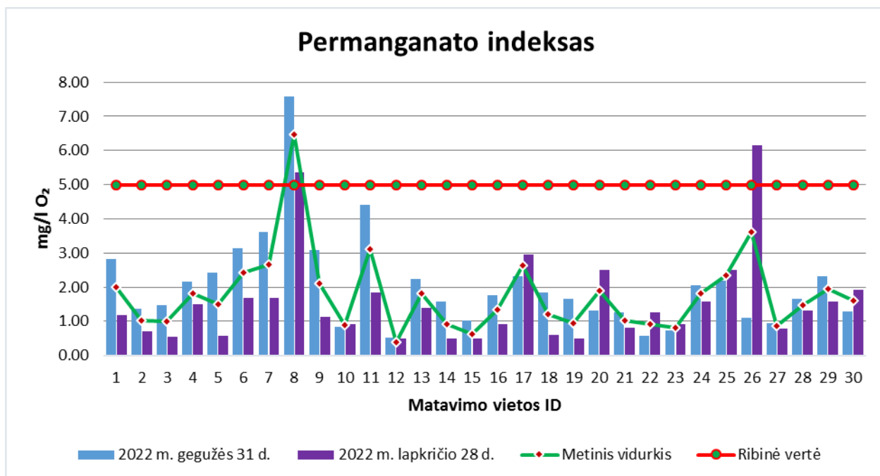
43 pav. Permanganato indekso koncentracijų vizualizacija Kupiškio rajono požeminiame vandenyje
