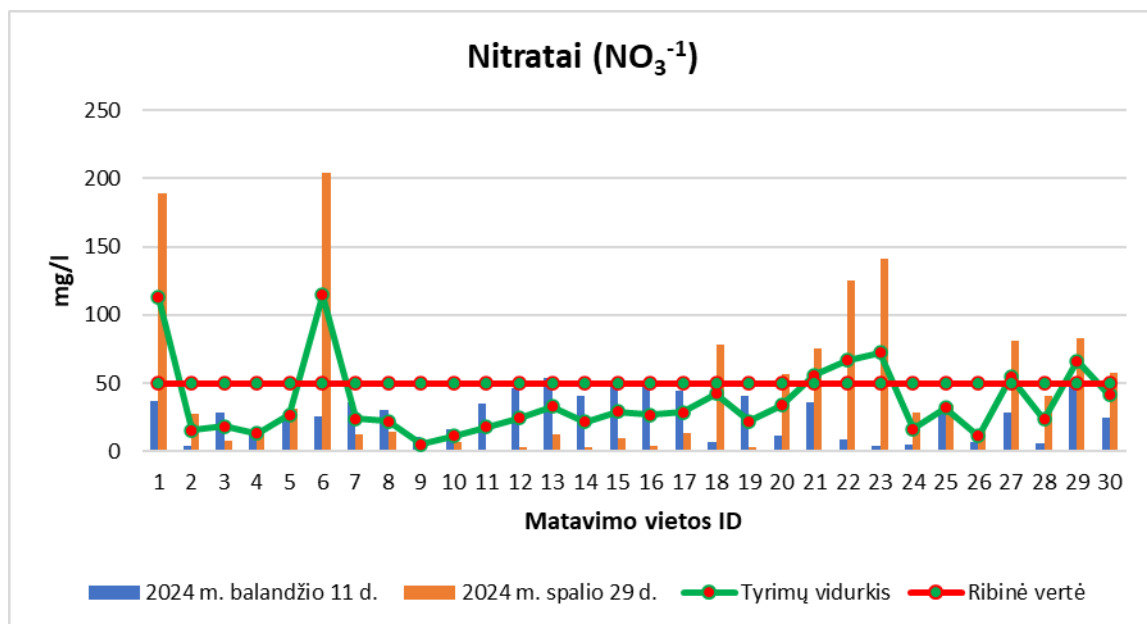
35 pav. Nitratų koncentracijų vizualizacija Kupiškio rajono požeminiame vandenyje
