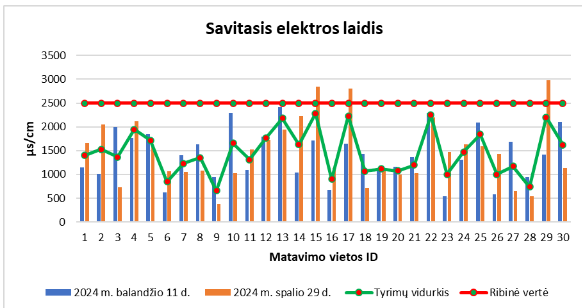
34 pav. Savitojo elektros laidžio koncentracijų vizualizacija Kupiškio rajono požeminiame vandenyje
