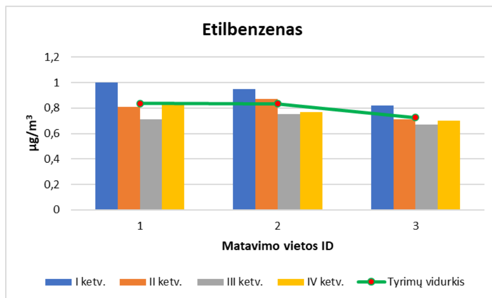
12 pav. Etilbenzeno koncentracijų pasiskirstymas Kupiškio rajone pagal matavimo vietos ID. (Ribinė vertė 20 \mu\text{g}/\text{m}^3 grafike neatvaizduojama, nes gautos etilbenzeno koncentracijos ženkliai mažesnės už ribinę vertę)
