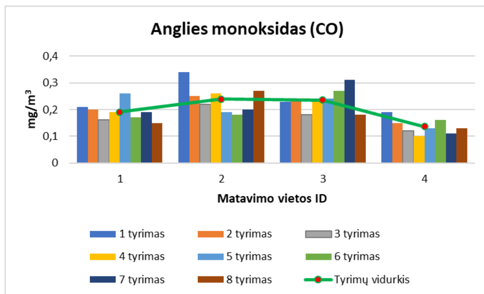
7 pav. CO koncentracijų pasiskirstymas Kupiškio rajone pagal matavimo vietos ID
