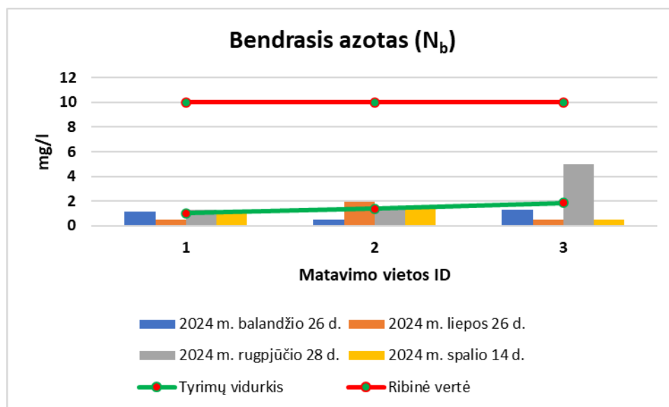
23 pav. Kupiškio rajono savivaldybės ežerų ir tvenkinio vandens N bendrojo tyrimų rezultatų vizualizacija. (Ribinė vertė 12 mg/l grafike neatvaizduojama, nes gautos N_b koncentracijos ženkliai mažesnės už ribinę vertę)
