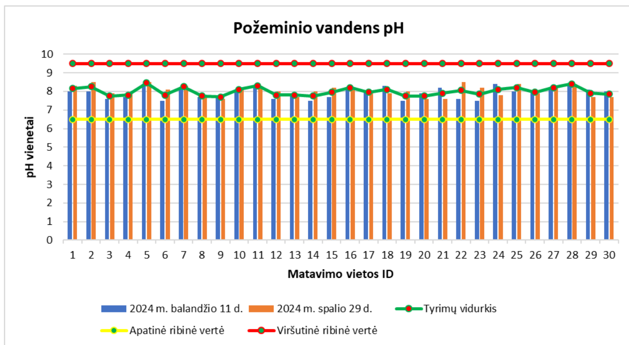
33 pav. pH koncentracijų vizualizacija Kupiškio rajono požeminiame vandenyje
