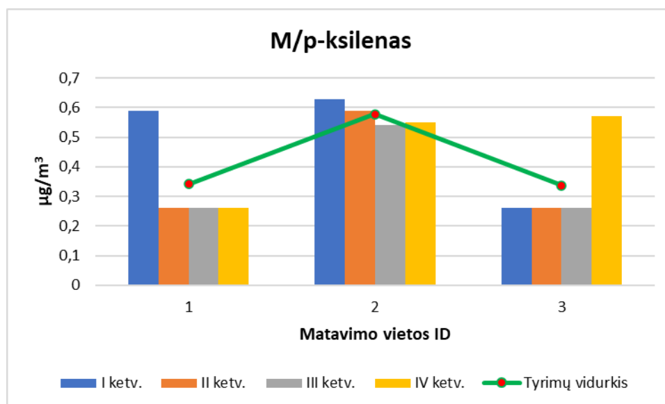
13 pav. m/p-ksileno koncentracijų pasiskirstymas Kupiškio rajone pagal matavimo vietos ID. (Ribinė vertė 200 \mu\text{g}/\text{m}^3 grafike neatvaizduojama, nes gautos m/p-ksileno koncentracijos ženkliai mažesnės už ribinę vertę)
