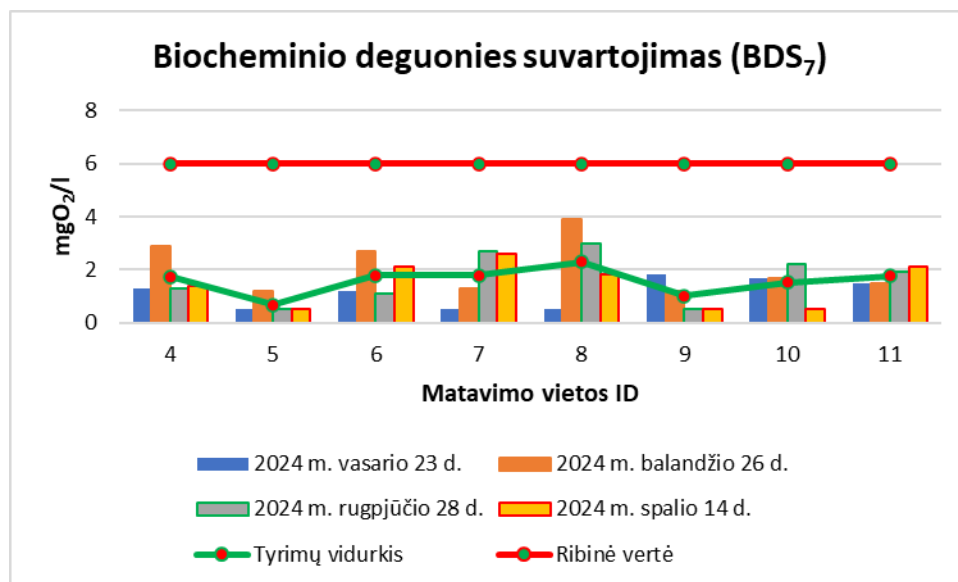
22 pav. Kupiškio rajono savivaldybės upių BDS 7 tyrimų rezultatų vizualizacija
