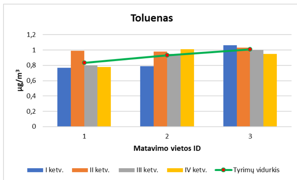
11 pav. Tolueno koncentracijų pasiskirstymas Kupiškio rajone pagal matavimo vietos ID. (Ribinė vertė 600 \mu\text{g}/\text{m}^3 grafike neatvaizduojama, nes gautos tolueno koncentracijos ženkliai mažesnės už ribinę vertę)
