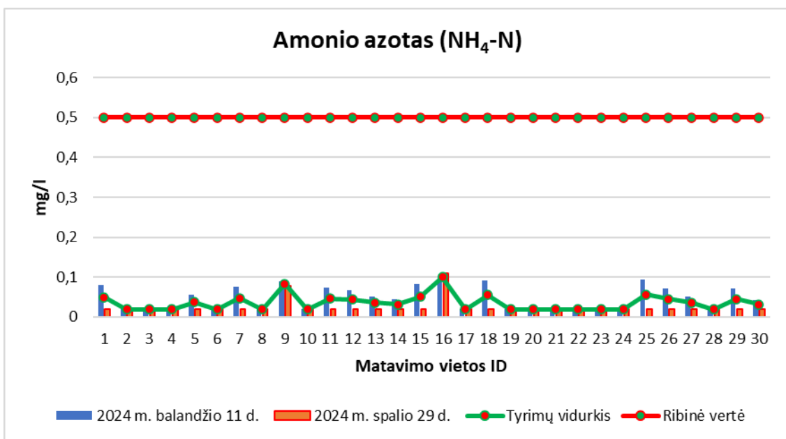
36 pav. Amonio azoto koncentracijų vizualizacija Kupiškio rajono požeminiame vandenyje
