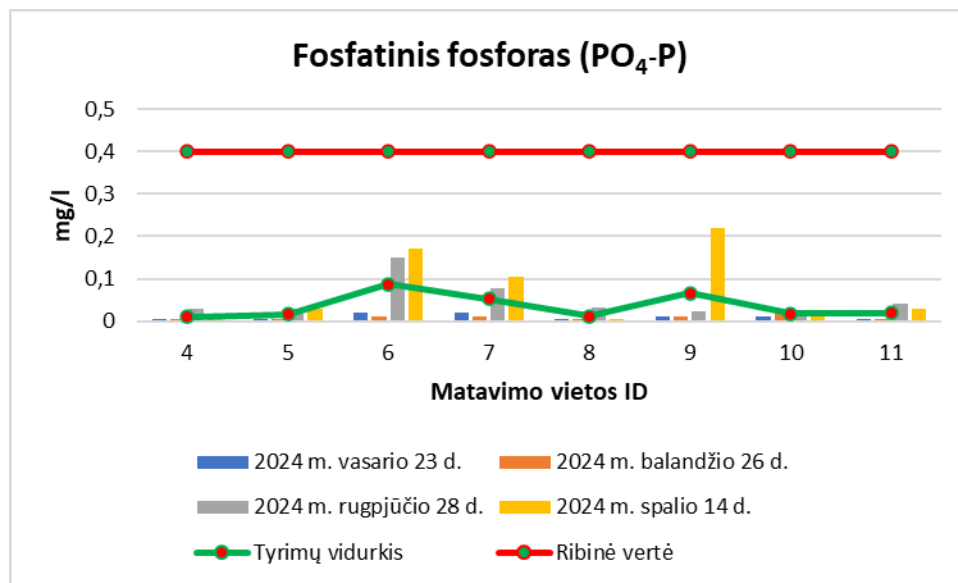
21 pav. Kupiškio rajono savivaldybės upių fosfatinio fosforo (PO 4 -P) tyrimų rezultatų vizualizacija
