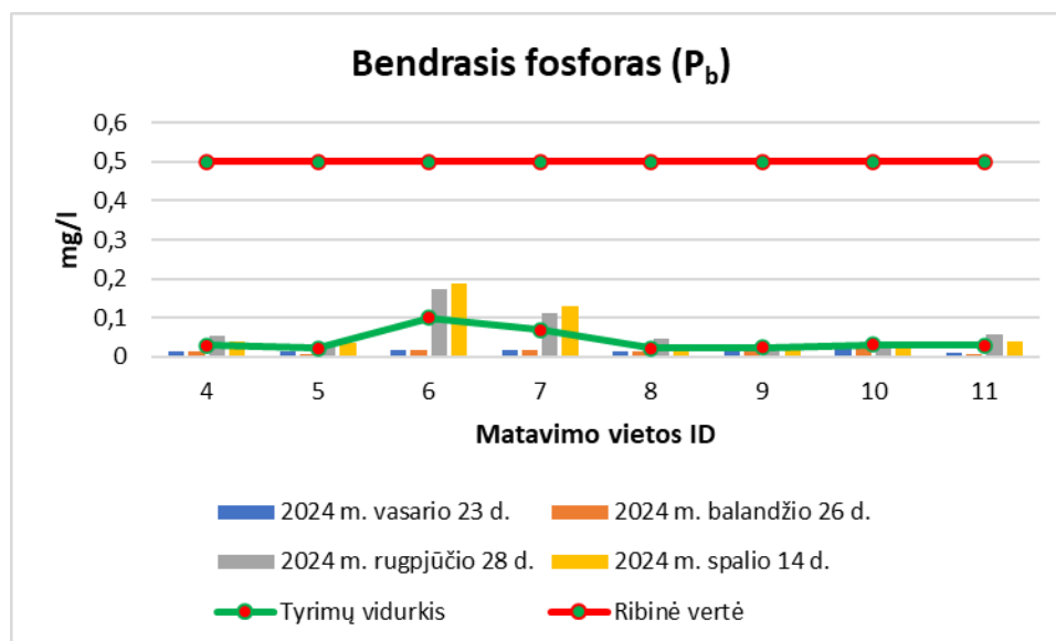
20 pav. Kupiškio rajono savivaldybės upių P bendrojo tyrimų rezultatų vizualizacija. (Ribinė vertė 1,6 mg/l grafike neatvaizduojama, nes gautos P b koncentracijos ženkliai mažesnės už ribinę vertę)
