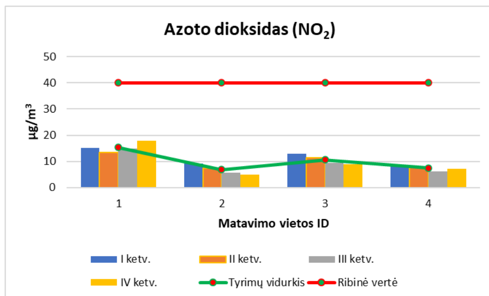
8 pav. NO 2 koncentracijų pasiskirstymas Kupiškio rajone pagal matavimo vietos ID
