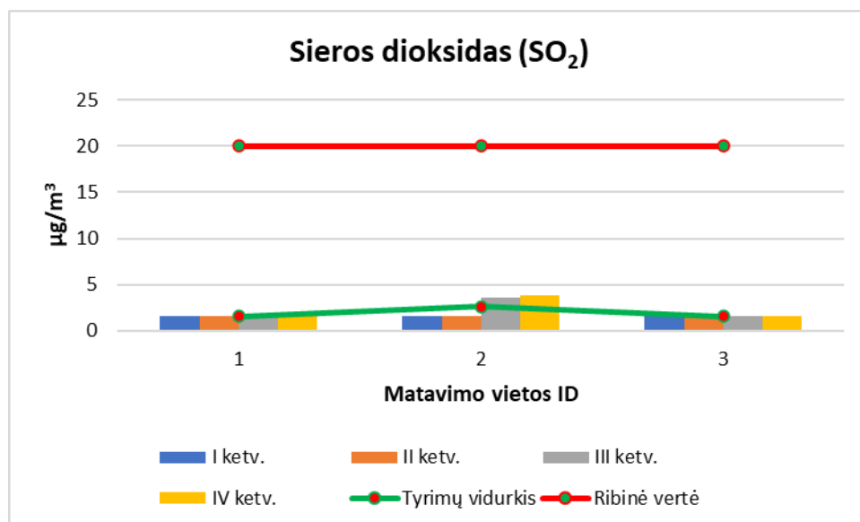
9 pav. SO 2 koncentracijų pasiskirstymas Kupiškio rajone pagal matavimo vietos ID
