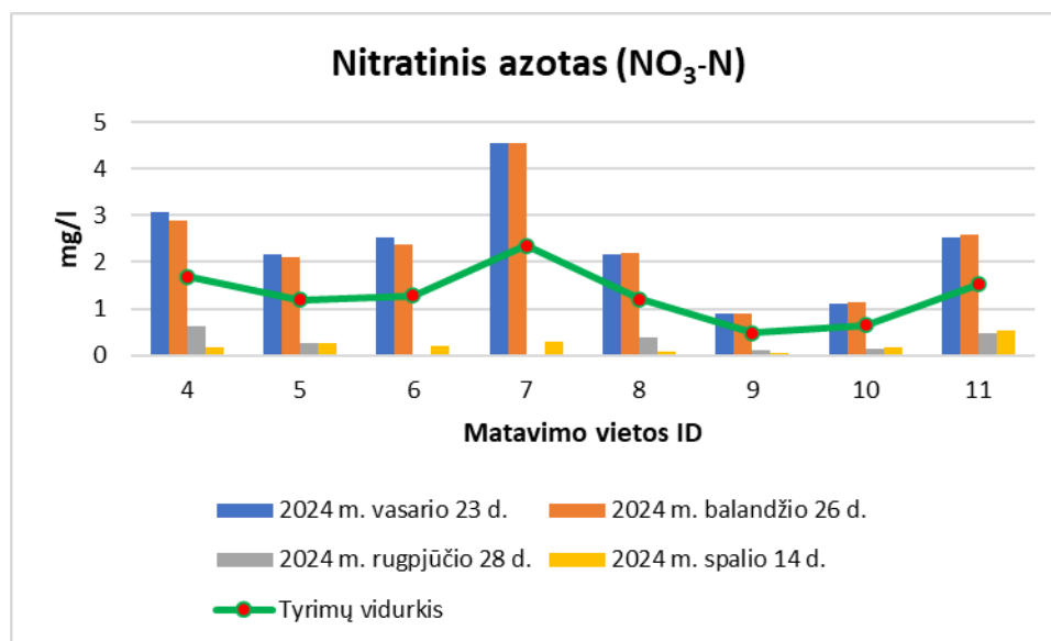
19 pav. Kupiškio rajono savivaldybės upių nitratinio azoto (NO 3 -N) tyrimų rezultatų vizualizacija. (Ribinė vertė 9 mg/l grafike neatvaizduojama, nes gautos NO 3 -N koncentracijos ženkliai mažesnės už ribinę vertę)
