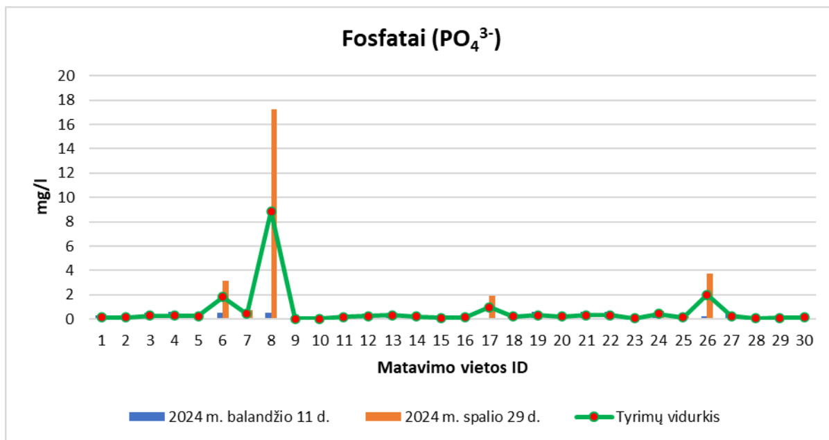
39 pav. Fosfatų koncentracijų vizualizacija Kupiškio rajono požeminiame vandenyje
