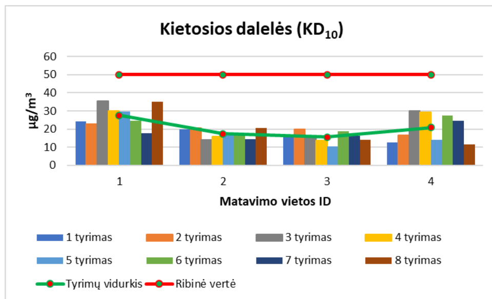
6 pav. KD 10 koncentracijų pasiskirstymas Kupiškio rajone pagal matavimo vietos ID
