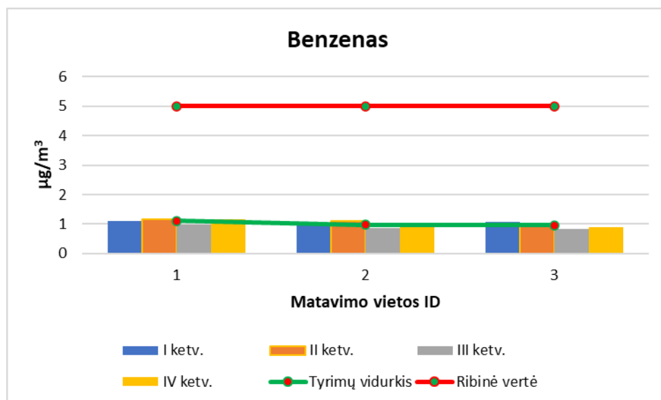
10 pav. Benzeno koncentracijų pasiskirstymas Kupiškio rajone pagal matavimo vietos ID
