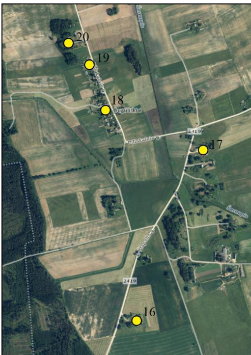
29 pav. Požeminio vandens tyrimo vietos Nr.16-20, Bugailiškių k., Šimonių sen. (šaltinis: sudaryta autorių maps.lt pagrindu)
