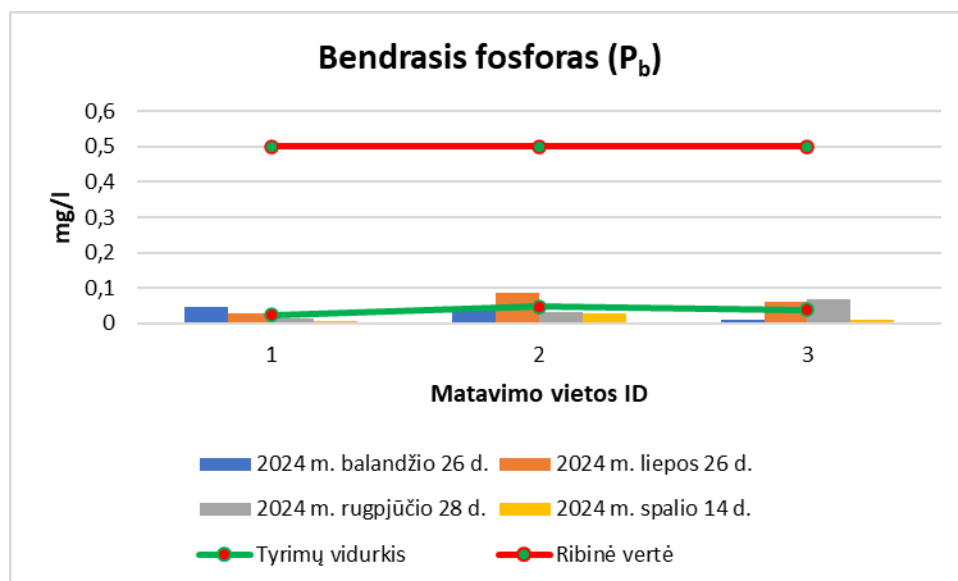
24 pav. Kupiškio rajono savivaldybės ežerų ir tvenkinio vandens P bendrojo tyrimų rezultatų vizualizacija. (Ribinė vertė 1,6 mg/l grafike neatvaizduojama, nes gautos P_b koncentracijos ženkliai mažesnės už ribinę vertę)
