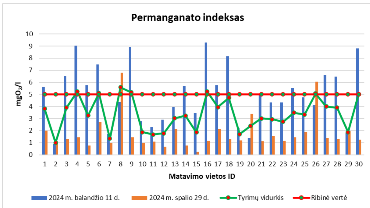
38 pav. Permanganato indekso koncentracijų vizualizacija Kupiškio rajono požeminiame vandenyje
