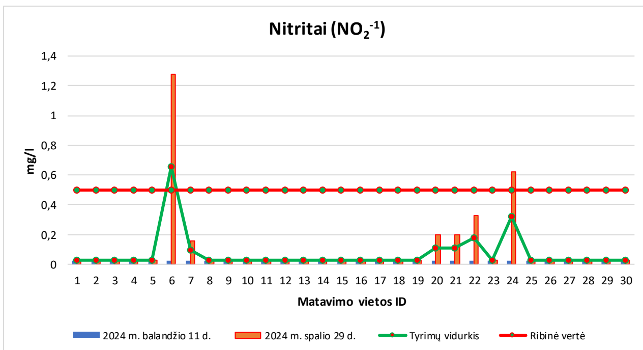
37 pav. Nitritų koncentracijų vizualizacija Kupiškio rajono požeminiame vandenyje
